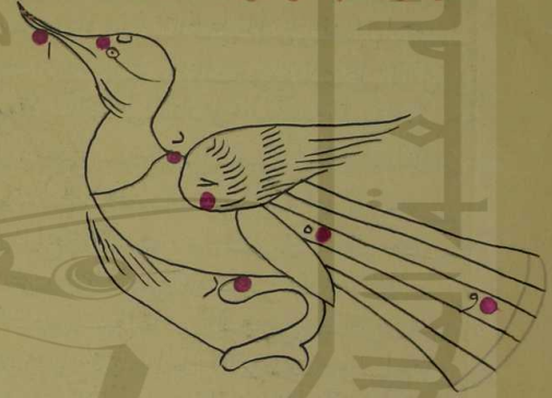
صورة كوكبة الغراب على ما يرى في السماء
